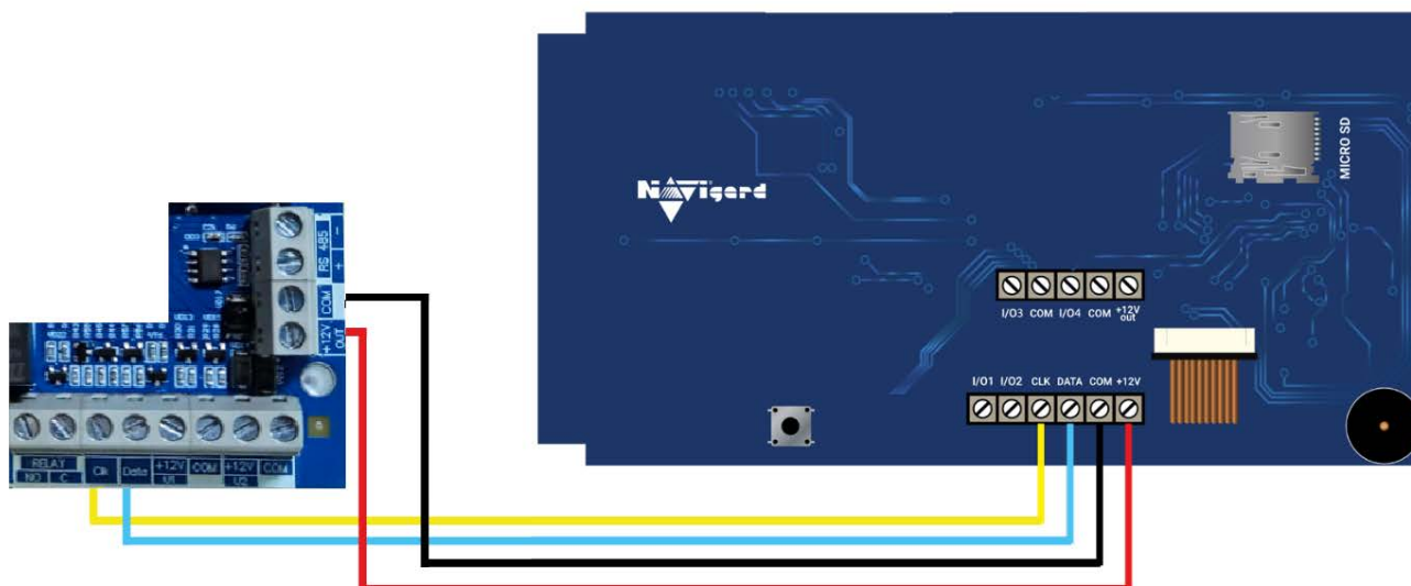
Рисунок 1. Пример подключения NV 8599 к ППО NV DG 2010 LED
